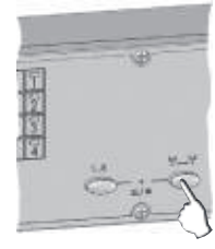
III. Zusätzlich Lerntaste am Funk-Temperaturaktor kurz drücken. (Bei abmelden eines Uhrensensors – Lerntaste innerhalb von 10 Sekunden nach Auslösen der Abmeldung am Uhrensensordrücken.)
