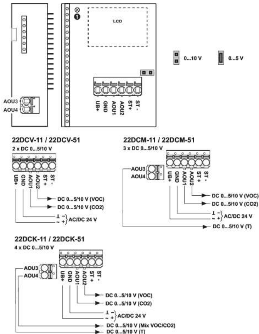
Aansluitschema voor 22DC...1, 22DTC...1
